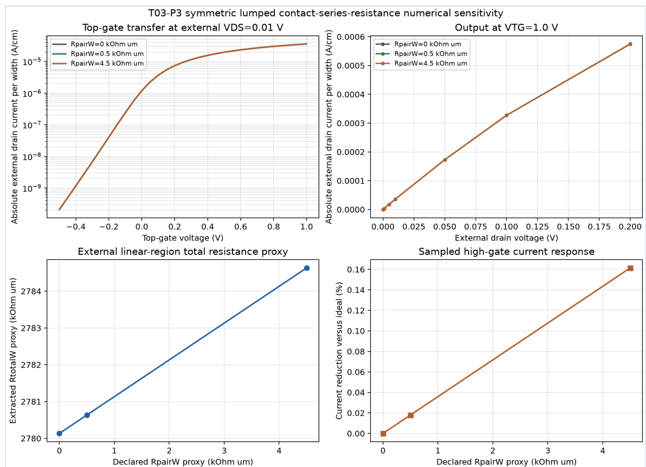
T03-P3 V2 接触电阻教学敏感性
