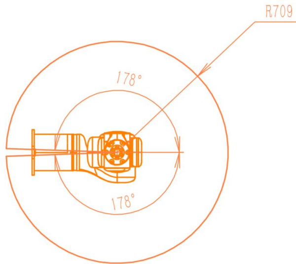
机器人可达空间示意图
