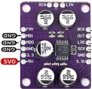
I2S ADC PCM 1808 (optional)
