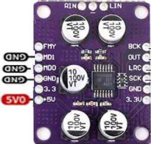
I2S ADC PCM 1808
