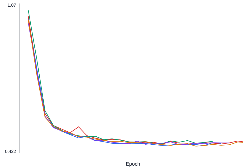
UNET
