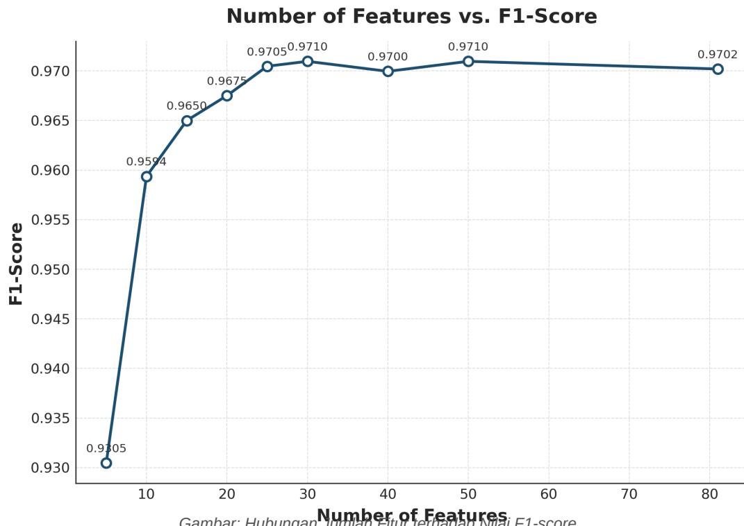
Gambar: Hubungan Jumlah Fitur terhadap Nilai F1-score
