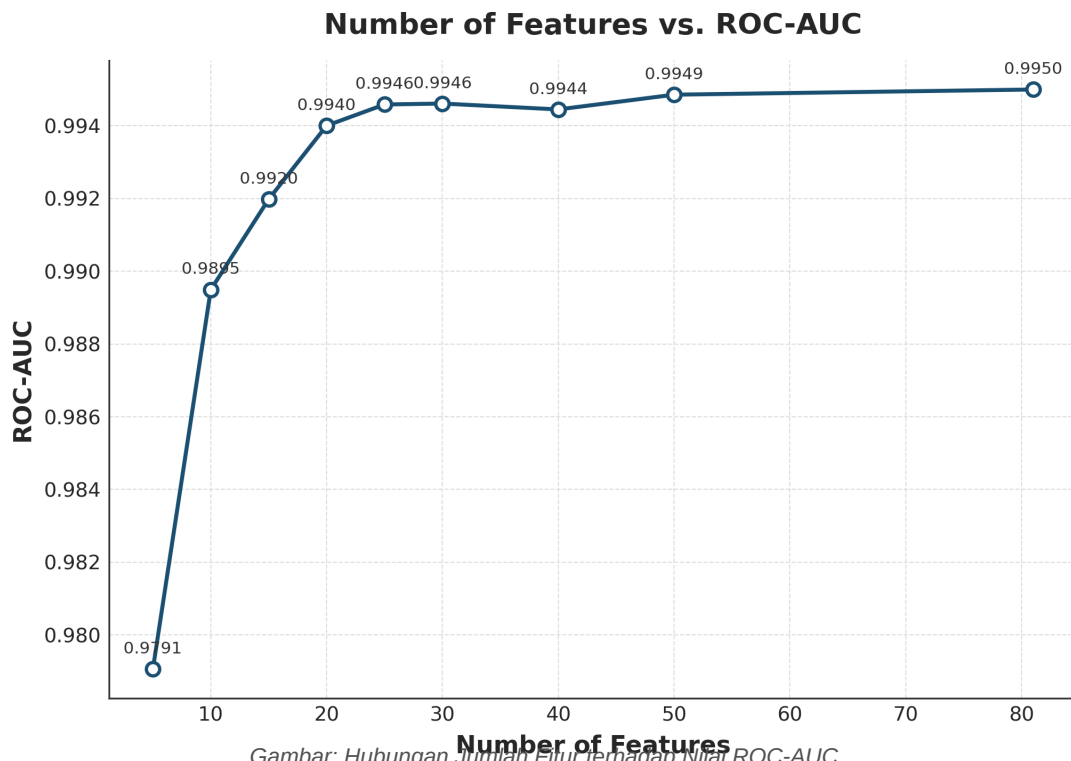
Gambar: Hubungan Jumlah Fitur terhadap Nilai ROC-AUC
