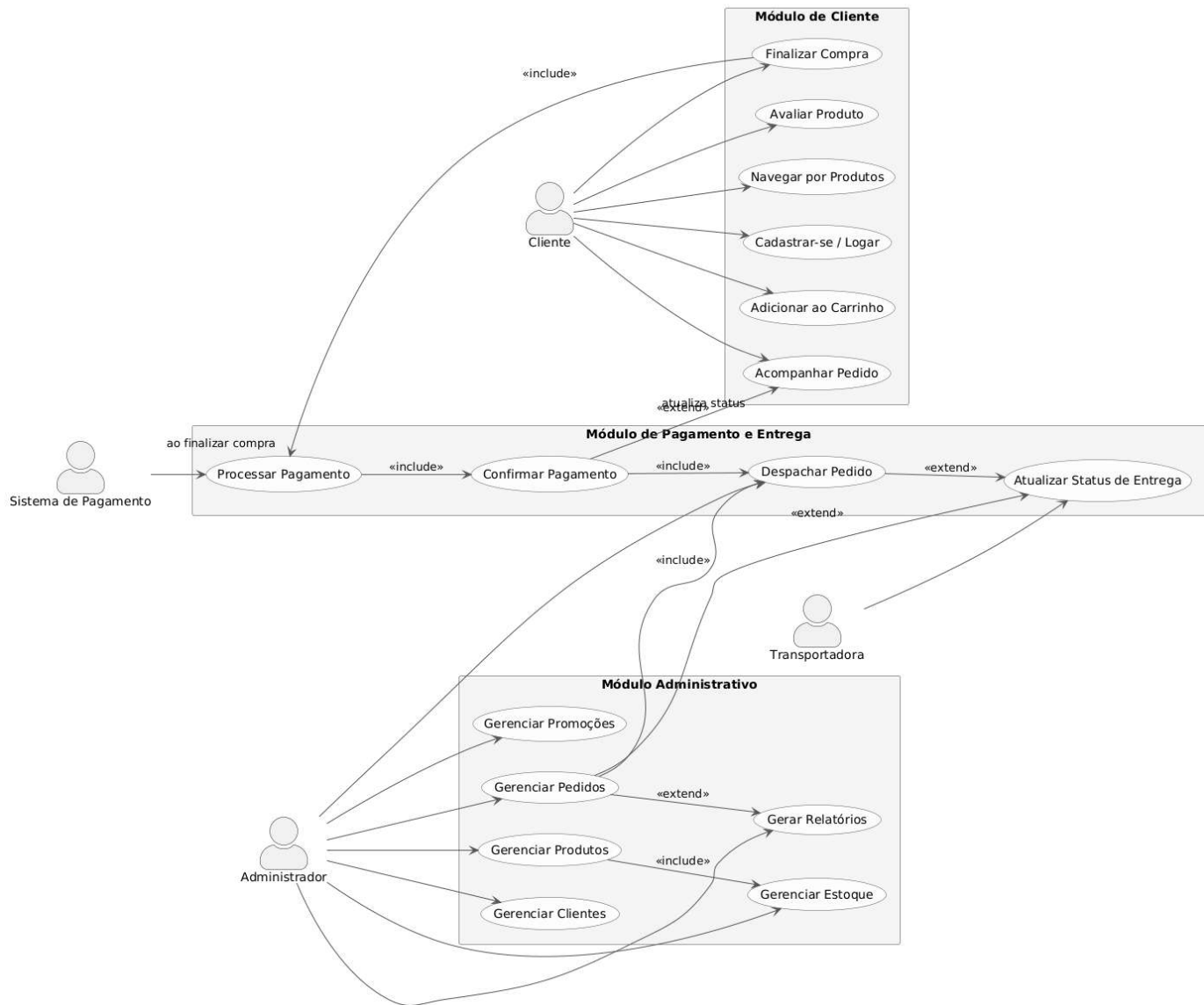
Diagrama de Casos de Uso - Sistema de E-commerce
