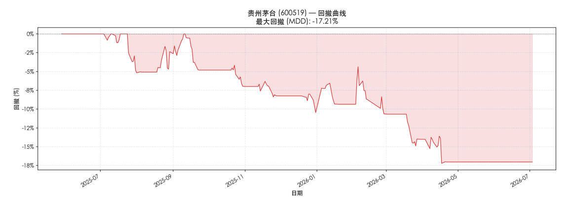
图 3：贵州茅台（600519）回撤曲线——MDD=-17.21%
