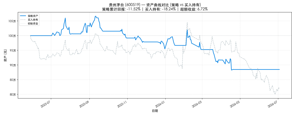
图 2：贵州茅台（600519）资产曲线对比——策略 vs 买入持有
