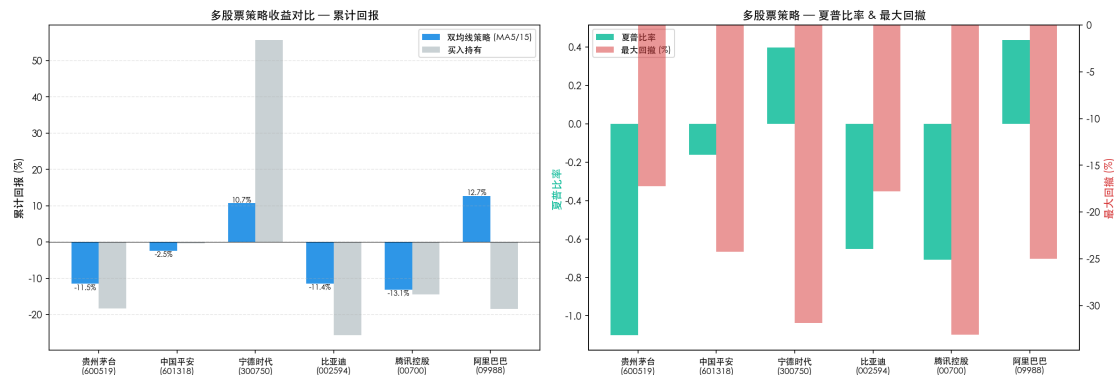
图 5：多股票双均线策略（MA5+MA15）回测对比——累计回报、夏普比率、最大回撤
