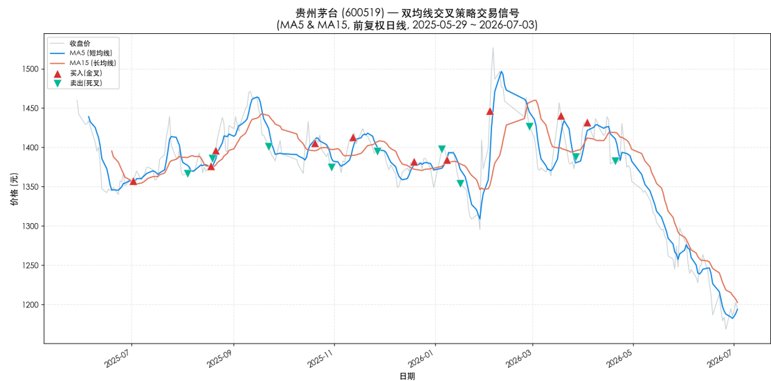
图 1：贵州茅台（600519）双均线策略交易信号（MA5 & MA15，红色▲买入，绿色▼卖出）
