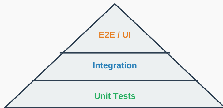
Abbildung 1: Die Test-Pyramide - Basis-Stabilität durch Unit Tests.
