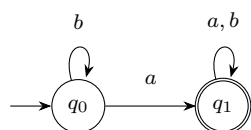
DFA pro slova obsahující aspoň jedno a .
