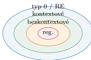
Chomského hierarchie jako vnořené třídy.
