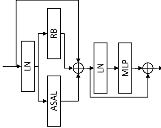
b) AWTRL 结构图
