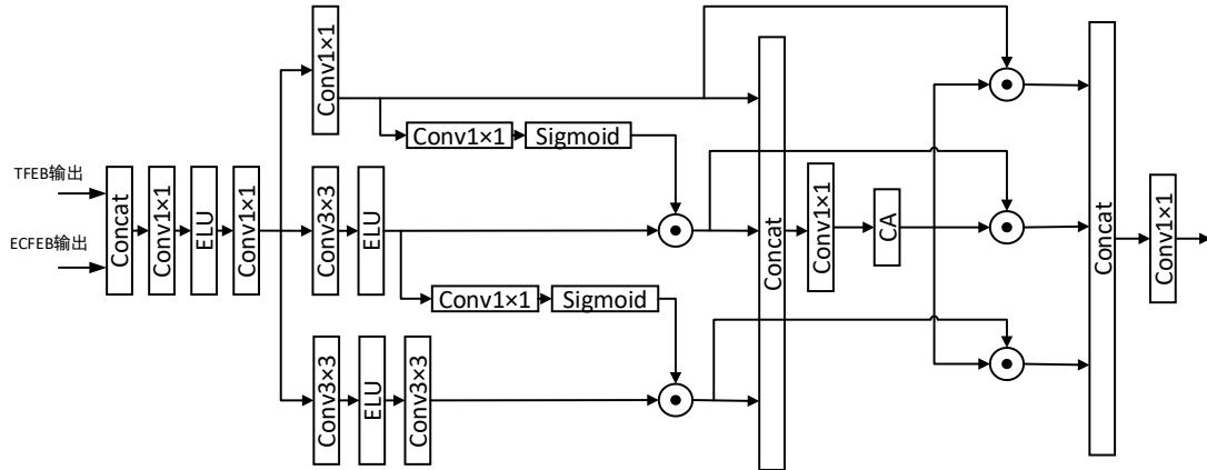
图 4-7 DFFB 模块的结构图
