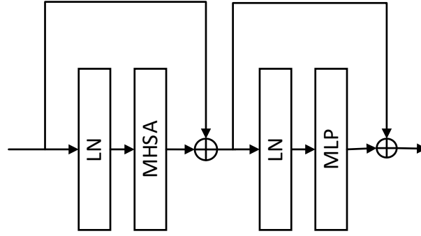
c) SWTL 结构图
