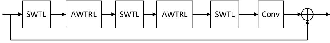
a) TFEB 总体结构图
