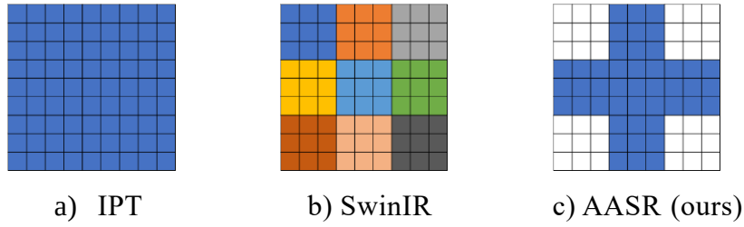
图 3-1 IPT、SwinIR 和 AASR 感受野比较
