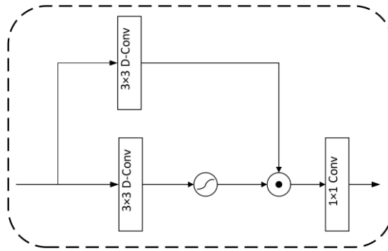
图 3-5 GDFN 结构图
