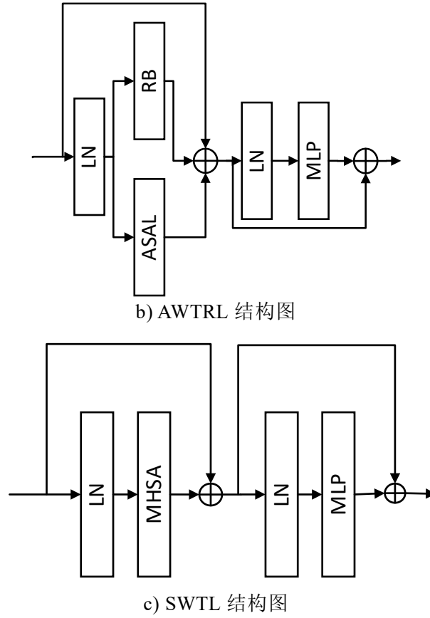
图 4-6 TFEB 模块及其子模块的结构图
