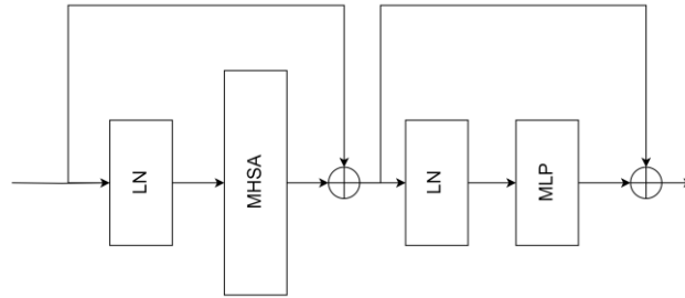
图 2-2 Transformer 块内部结构
