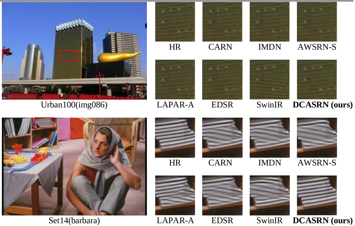
图 4-9 DCASRN 与其他方法主观视觉效果
