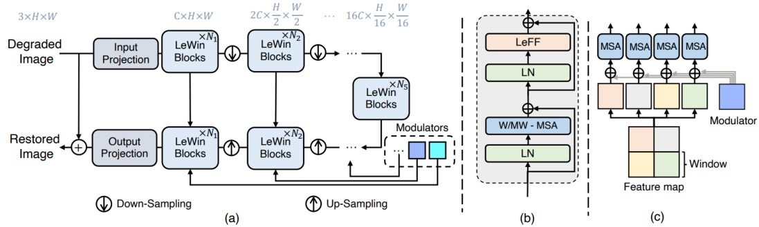
图 2-9 Uformer 网络结构图 [47]
