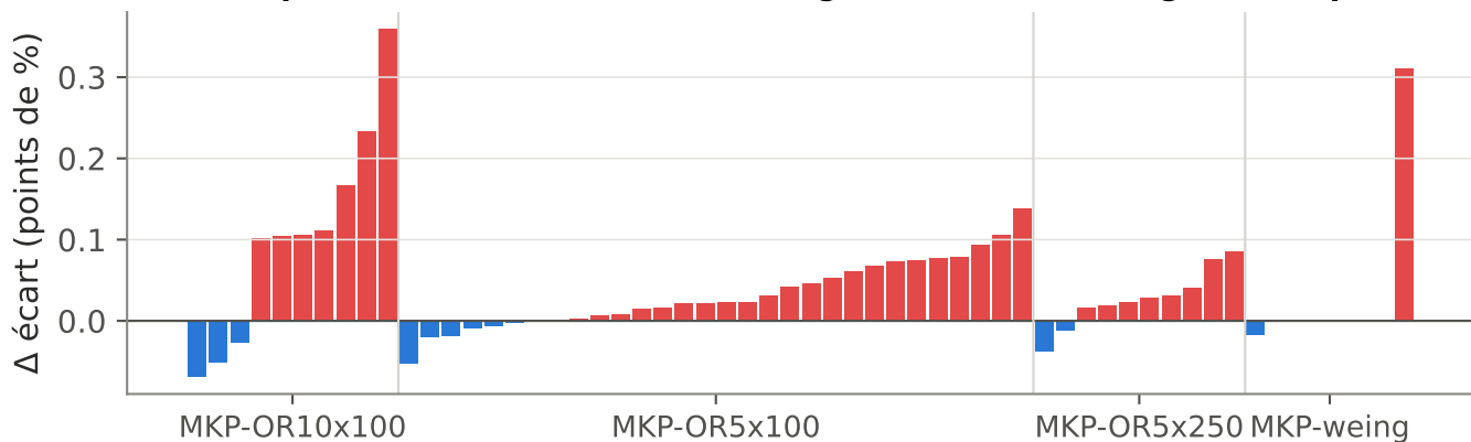
AG + QL pré-entraîné vs Meilleure config. fixe (oracle) : 12 gains, 39 pertes
