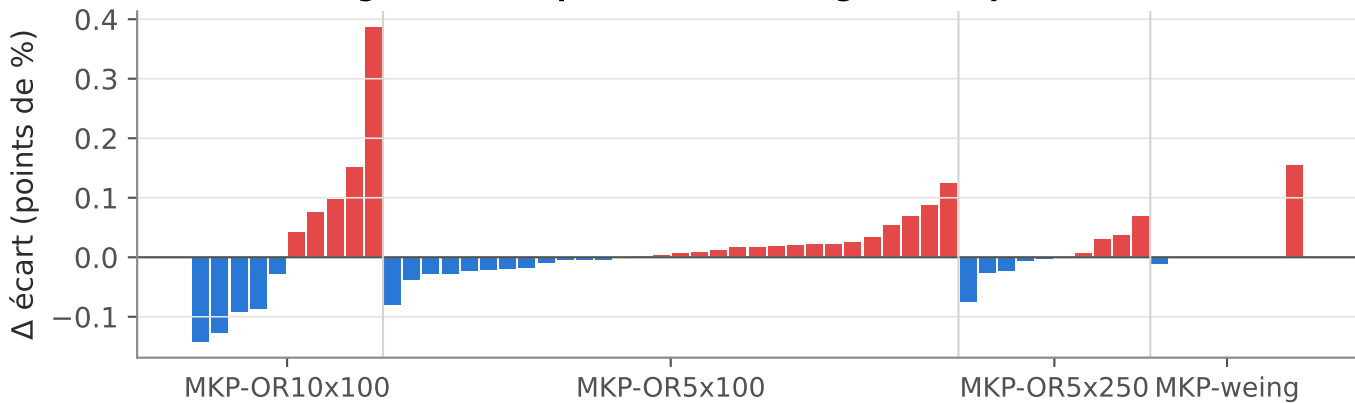
AG + QL (en ligne) vs AG op. aléatoires : 25 gains, 27 pertes
