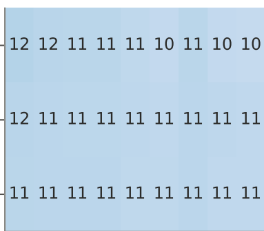
UCB1 · SC
