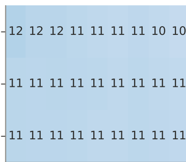
UCB1 · ASC
