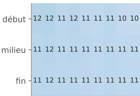
UCB1 · UC
