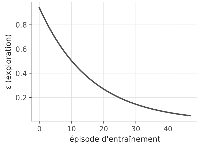
Décroissance de l'exploration
