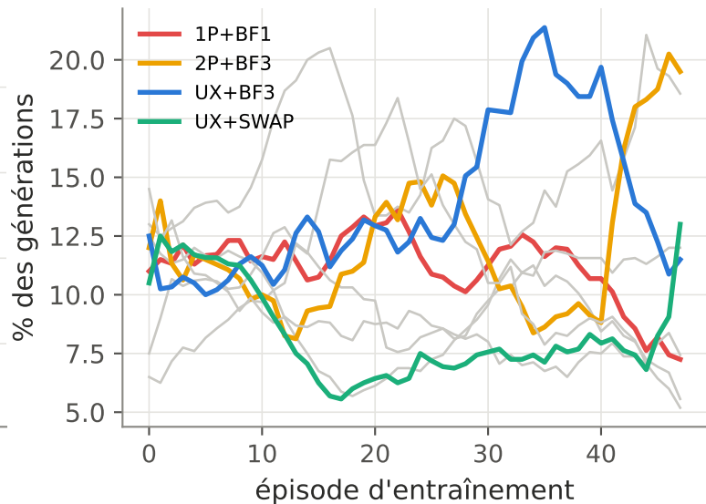
Part de chaque action (moyenne glissante ; gris : autres)
