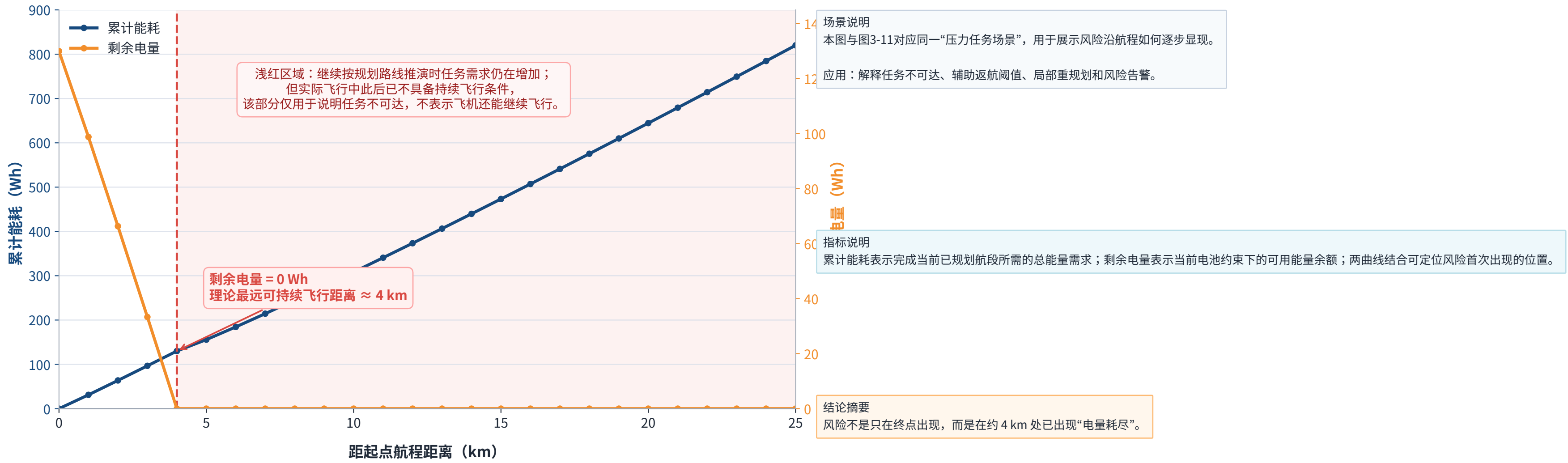
图3-12 沿航程累计能耗与剩余电量变化图
