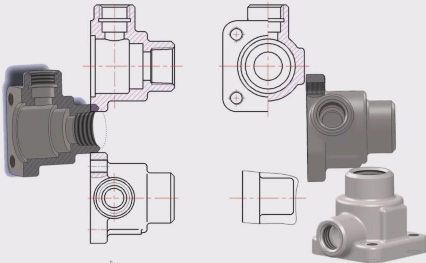
阀体1零件图
