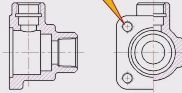
阀体1零件图
