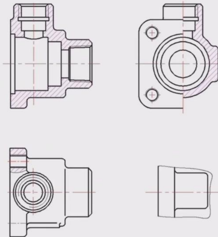
阀体1零件图
