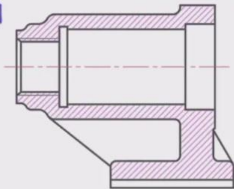
泵体视图
