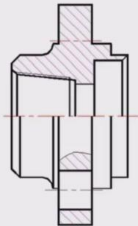
阀体接头2零件图
