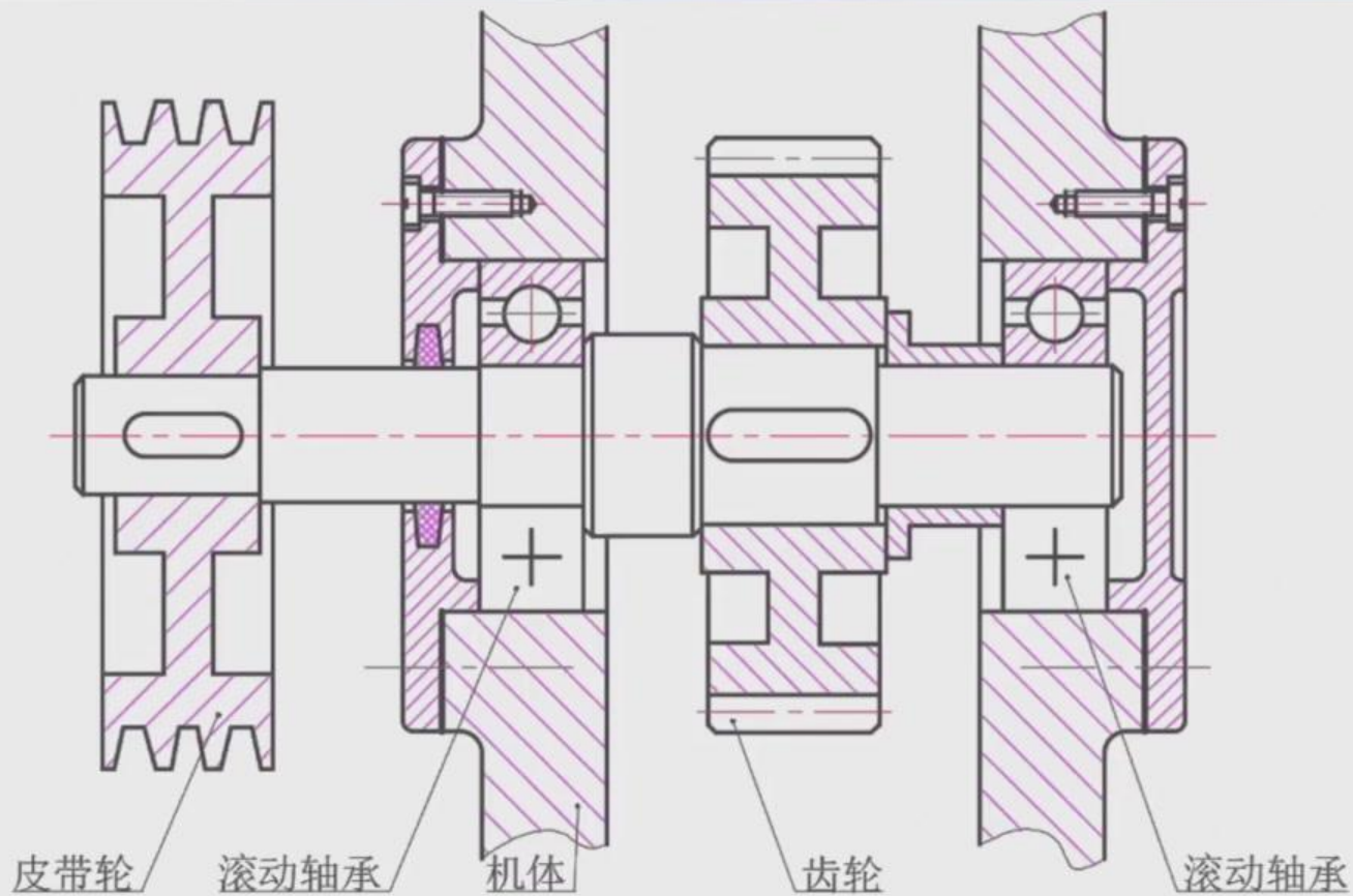
轴系结构设计方案一
