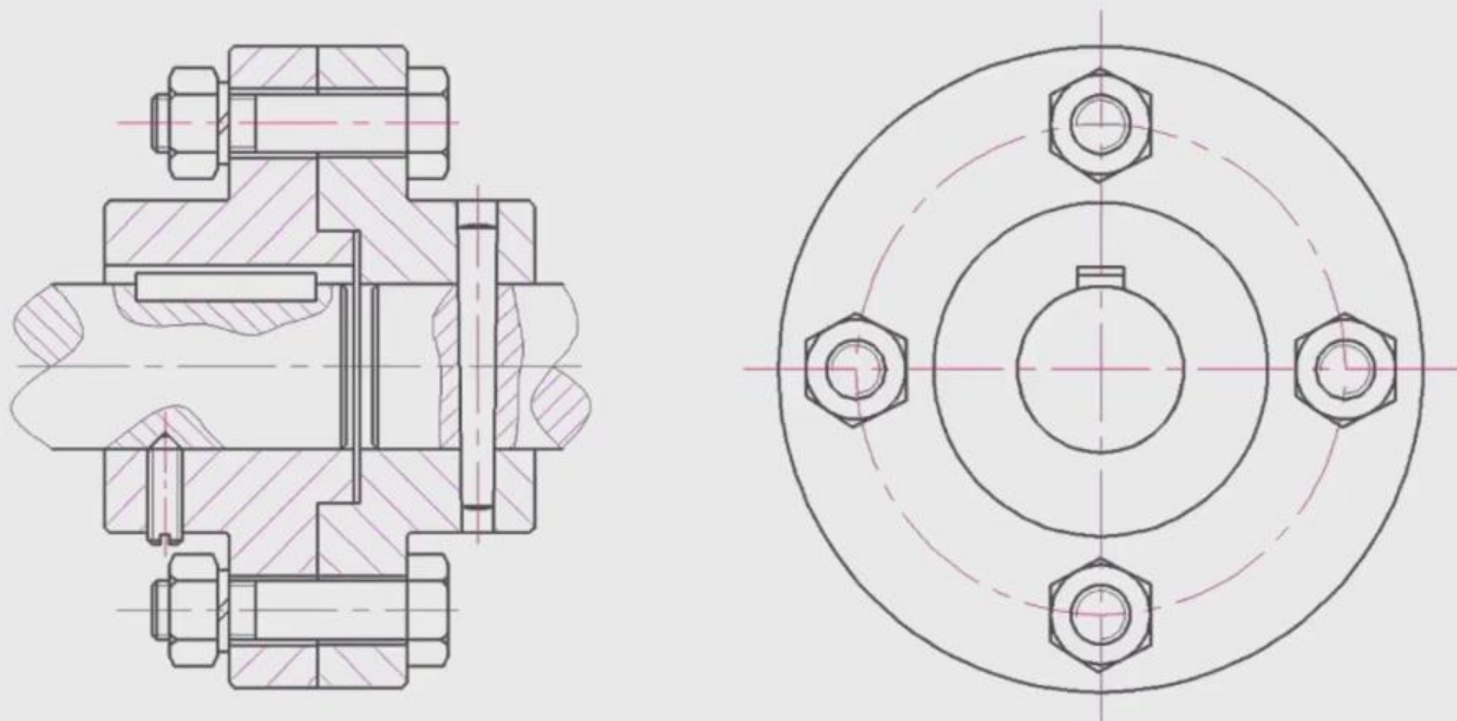
正确的联轴器装配图
