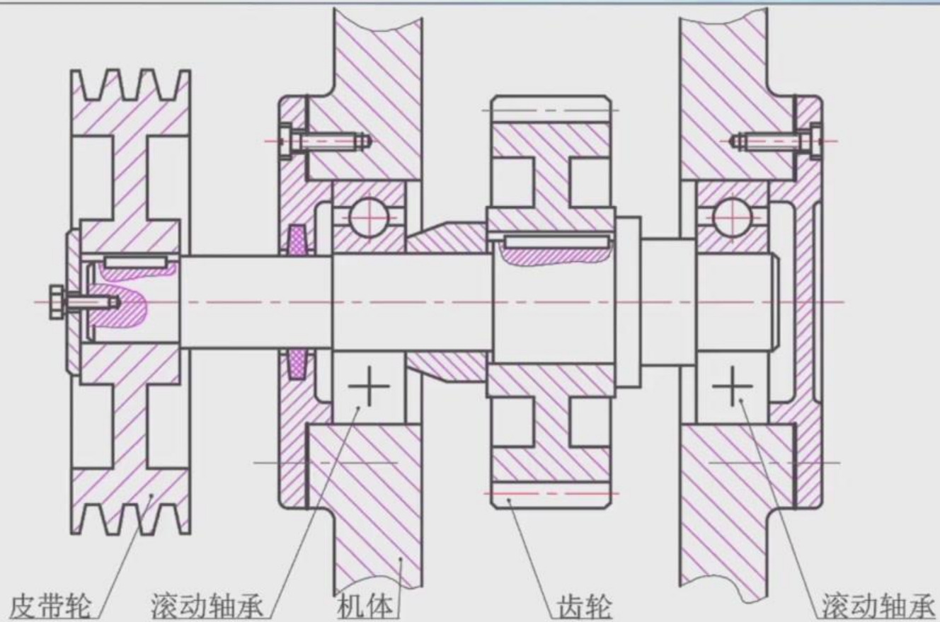
轴系结构设计方案二
