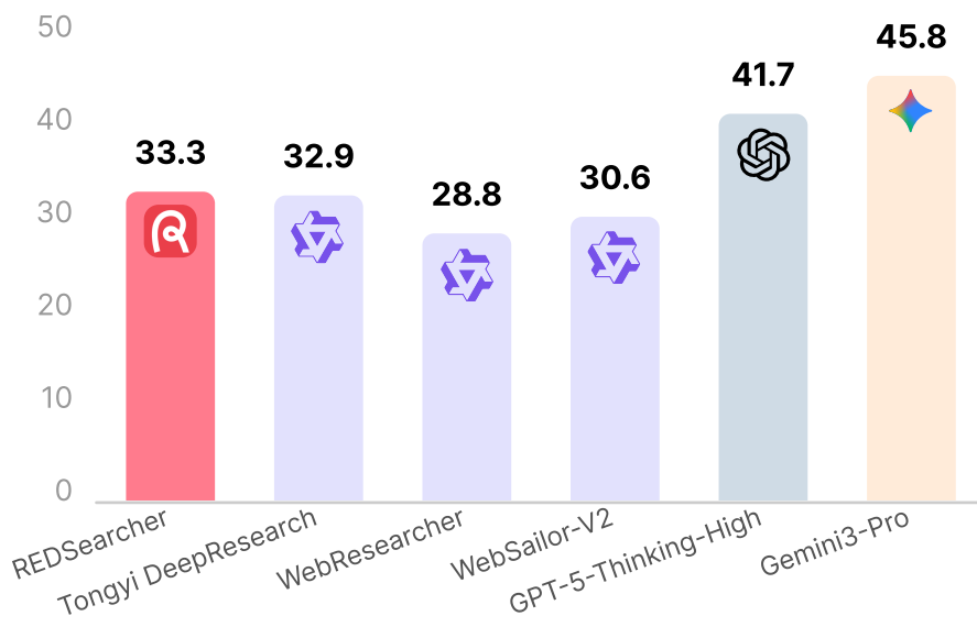
HLE
