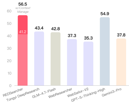
HLE
