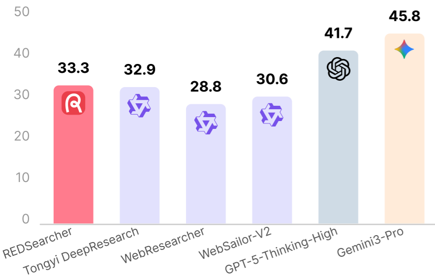
HLE
