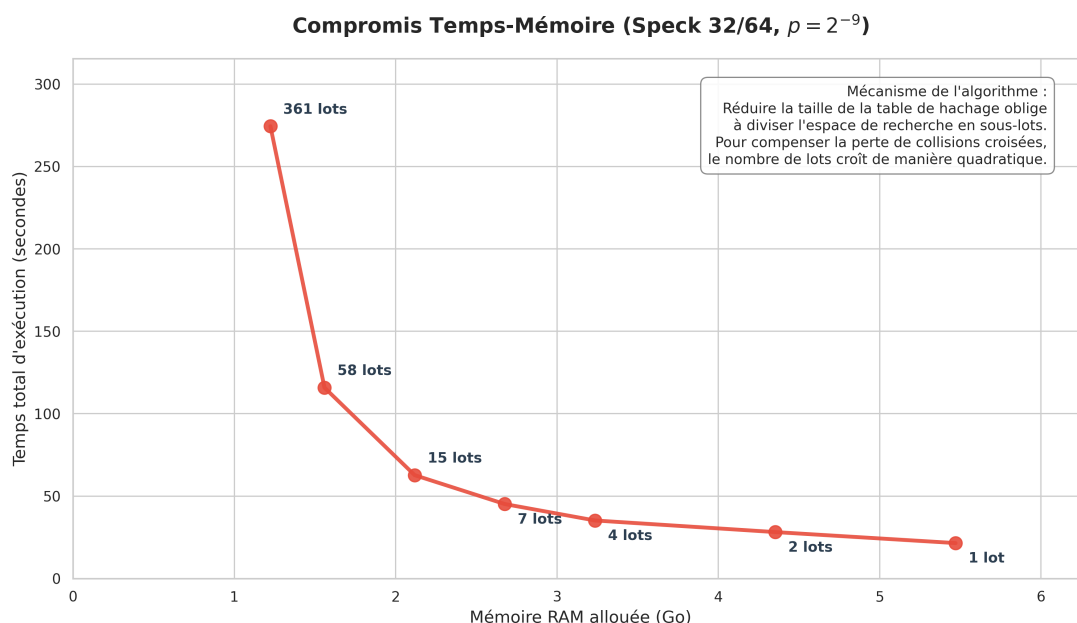
Figure 4 – Courbe du compromis Temps-Mémoire sur Speck 32/64. La réduction de la RAM disponible contraint l'algorithme à multiplier les lots d'évaluation, entraînant une hausse du temps d'exécution.
