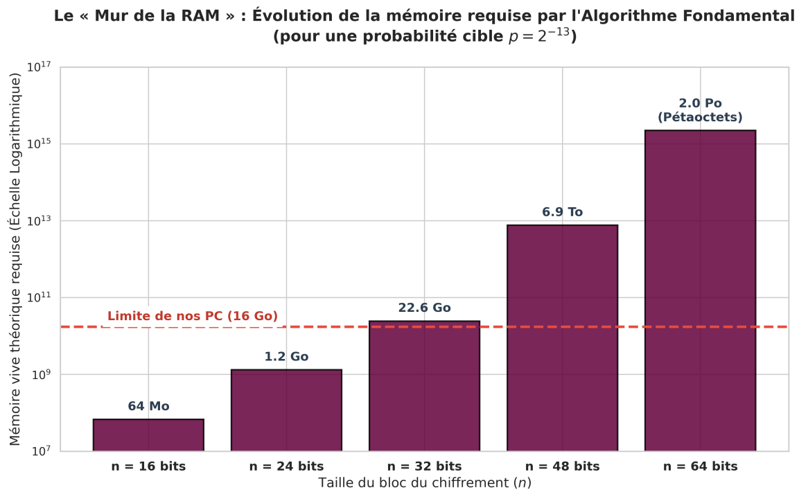
Figure 3 – L’explosion combinatoire de la mémoire : le « mur de la RAM ». Dès n = 32 , l’algorithme fondamental pur dépasse les capacités d’un ordinateur personnel standard. Pour n = 64 , il outrepassé les capacités des plus grands supercalculateurs mondiaux.
