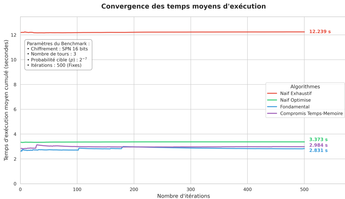
Figure 2 – Évolution de la convergence des temps moyens d'exécution pour les variantes de recherche différentielle (SPN 16 bits, exécution séquentielle stricte). La stabilisation des courbes valide l'application de la loi des grands nombres sur cet échantillon.
