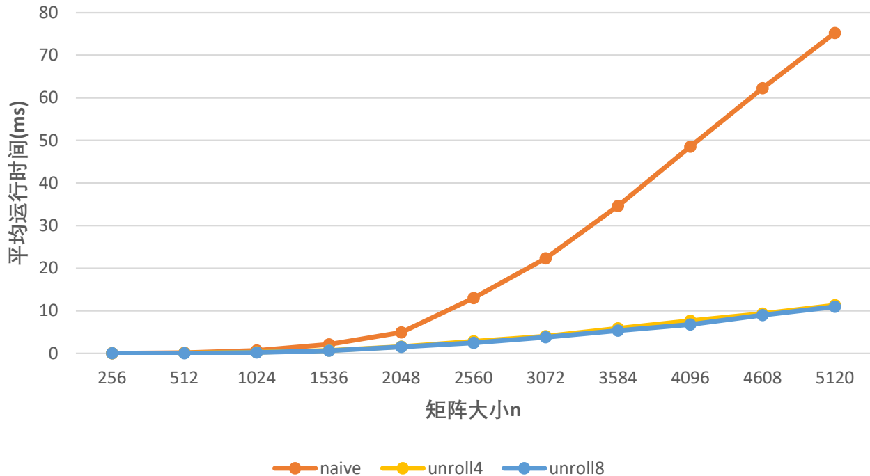
naive 算法与循环展开优化算法对比
