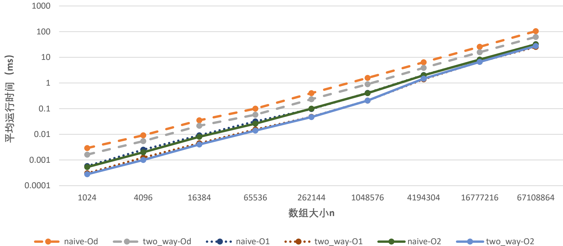
编译器优化力度对性能的影响(二)
