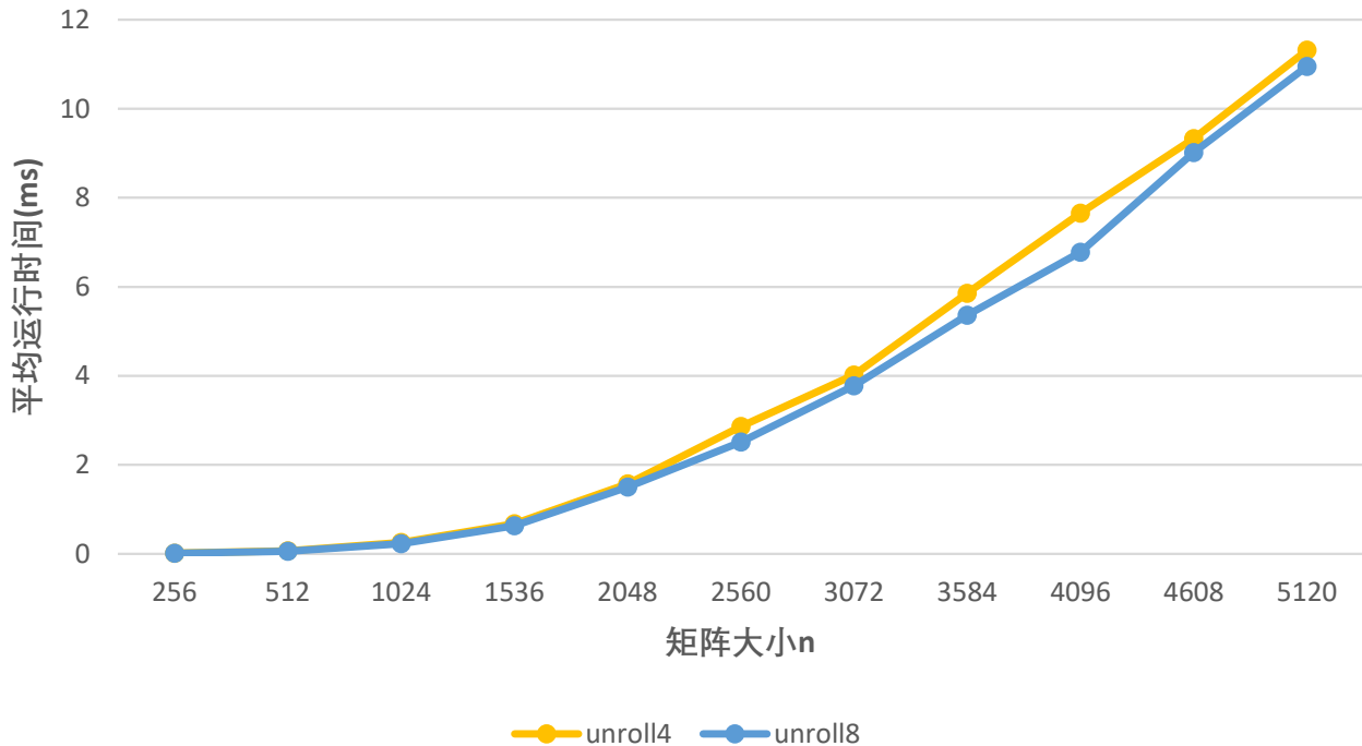
四路展开与八路展开优化算法对比
