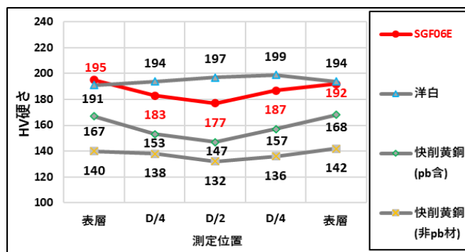
HV硬さ
