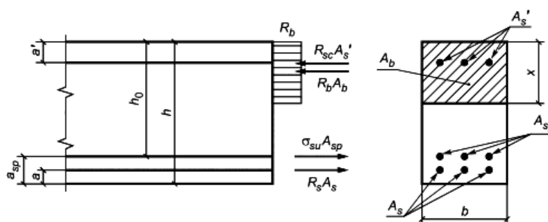
Рисунок М.1 - Схема усилий и напряжений в сечении, нормальном к продольной оси изгибаемого предварительно напряженного элемента без сцепления арматуры с бетоном, при его расчете по
