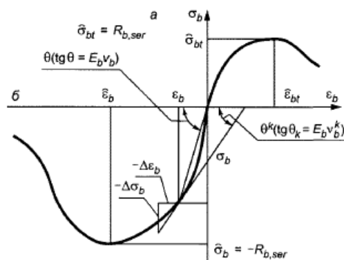
Рисунок Г.1 - Криволинейные диаграммы деформирования бетона
