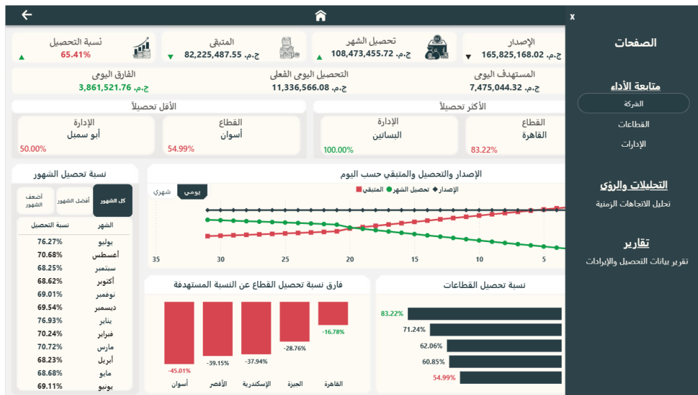
Page-navigation menu.
