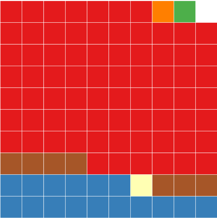
Assemblage 4 (n=25)
