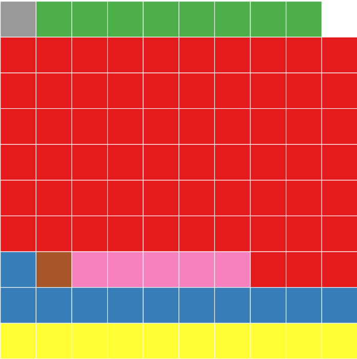
Assemblage 6 (n=24)
