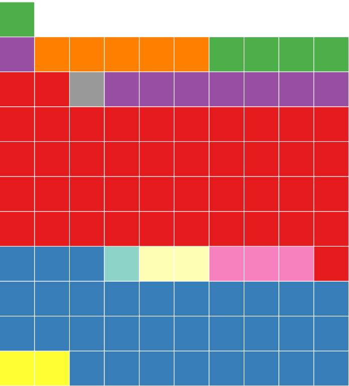
Assemblage 5 (n=27)
