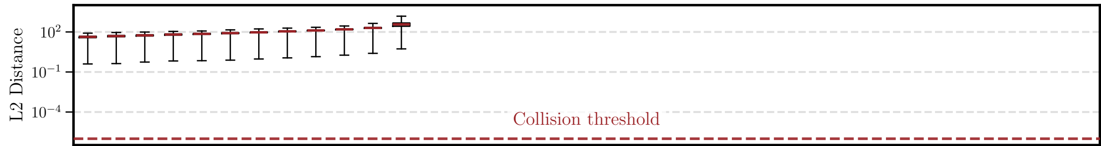
gpt2
