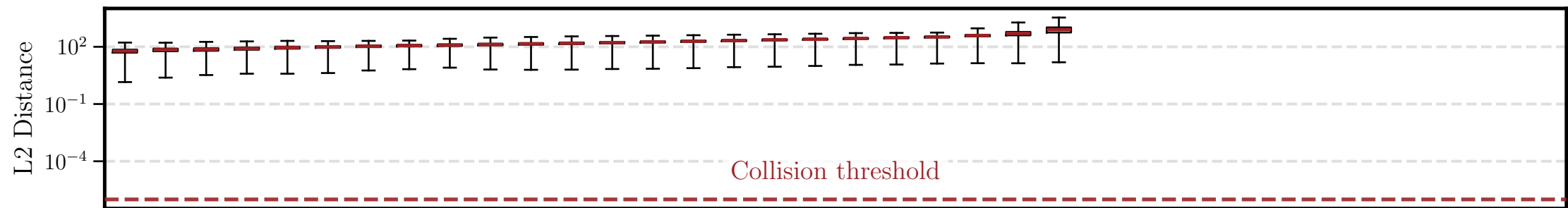
gpt2-medium
