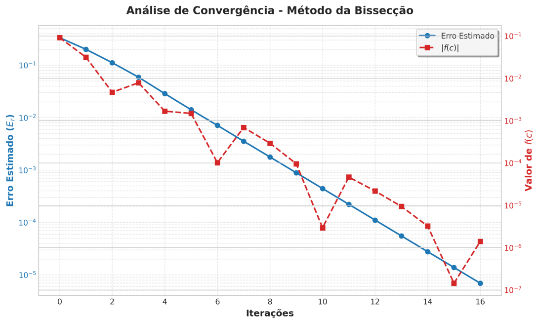
Figura 1: Gráfico de convergência do erro relativo e magnitude da função f_1(T) pelo Método da Bissecção.
