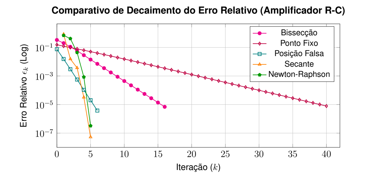
Figura 1.15: Superposição vetorial das taxas de convergência. O contraste entre a reta longa do Ponto Fixo ( \mathcal{O}(N) ) e a inflexão abrupta (concavidade para baixo) do Método de Newton reflete geometricamente as distintas ordens assintóticas.
