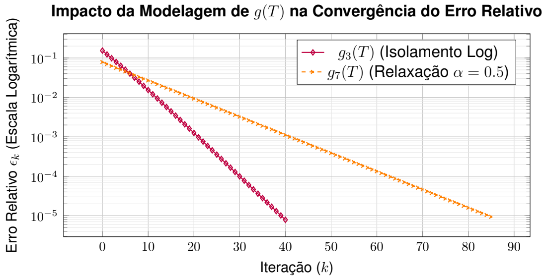
Figura 1.7: Comparativo das taxas de convergência para T_{0.1} usando g_3(T) e g_7(T) .
