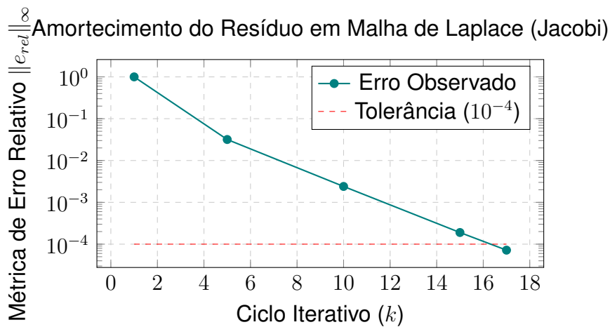
Figura 2.3: Amortecimento do Resíduo em Malha de Laplace (Jacobi)
