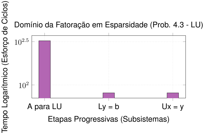
Figura 2.2: Domínio da Fatoração em Esparsidade (Prob. 4.3 - LU)
