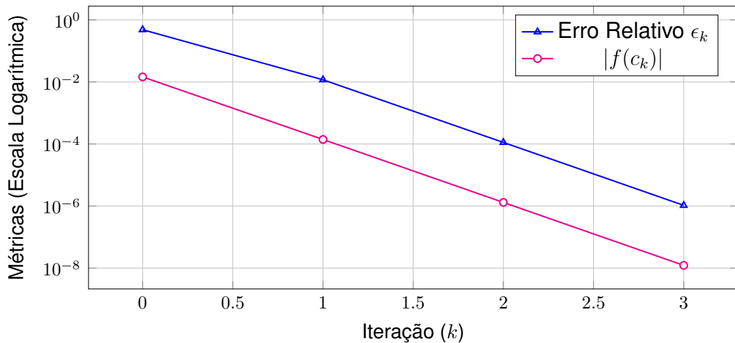
Figura 1.5: Gráfico de convergência da aproximação do ângulo de lançamento \alpha pelo Método da Posição Falsa. A queda abrupta nas primeiras iterações valida o alto desempenho da interpolação linear frente à topologia da função analisada.
