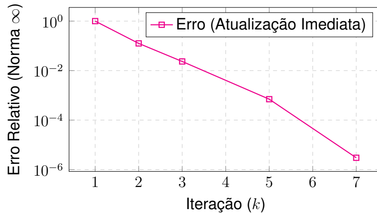
Decaimento de Convergência Acelerada - Gauss-Seidel
