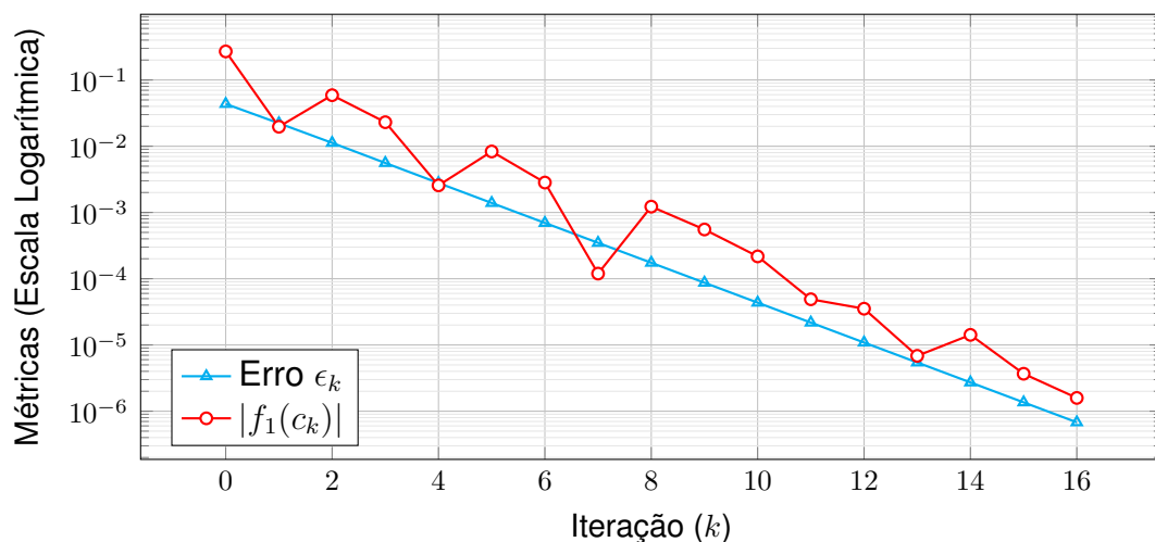
Figura 1.3: Convergência do erro na determinação da taxa (Plano A).
