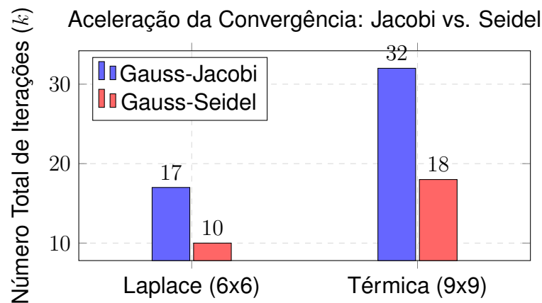
Figura 2.5: Aceleração da Convergência: Jacobi vs. Seidel
