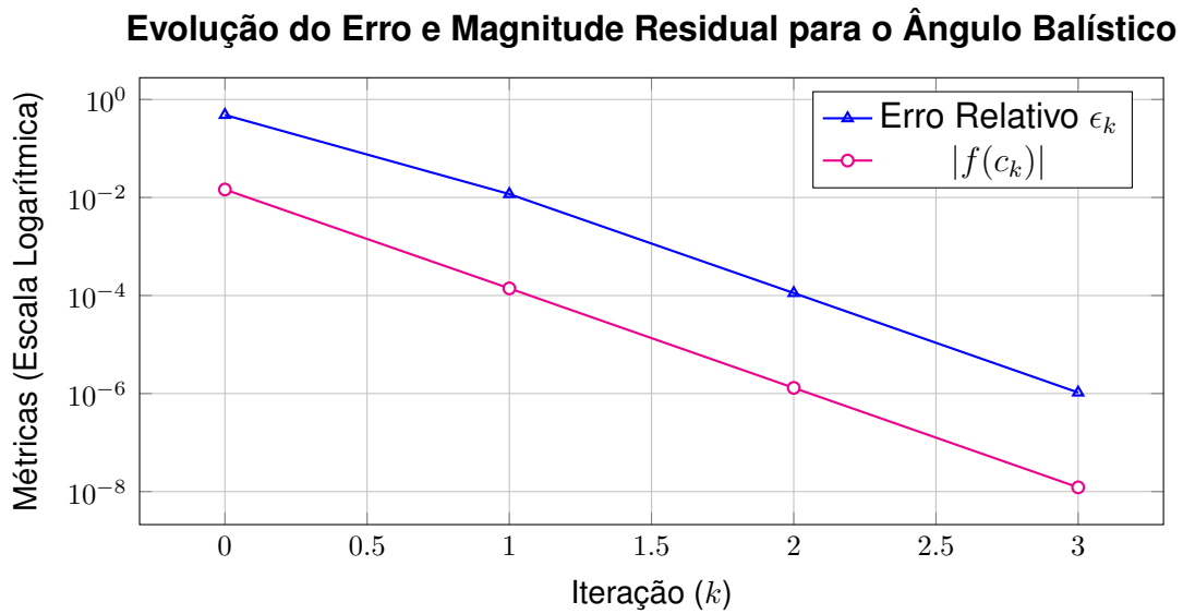
Figura 1.5: Convergência iterativa da Posição Falsa na busca de \alpha .
