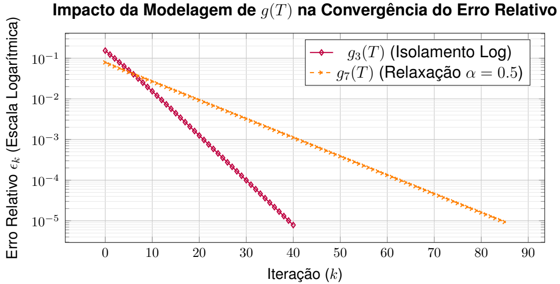
Figura 1.7: Comparativo das taxas de convergência para T_{0.1} usando g_3(T) e g_7(T) .
