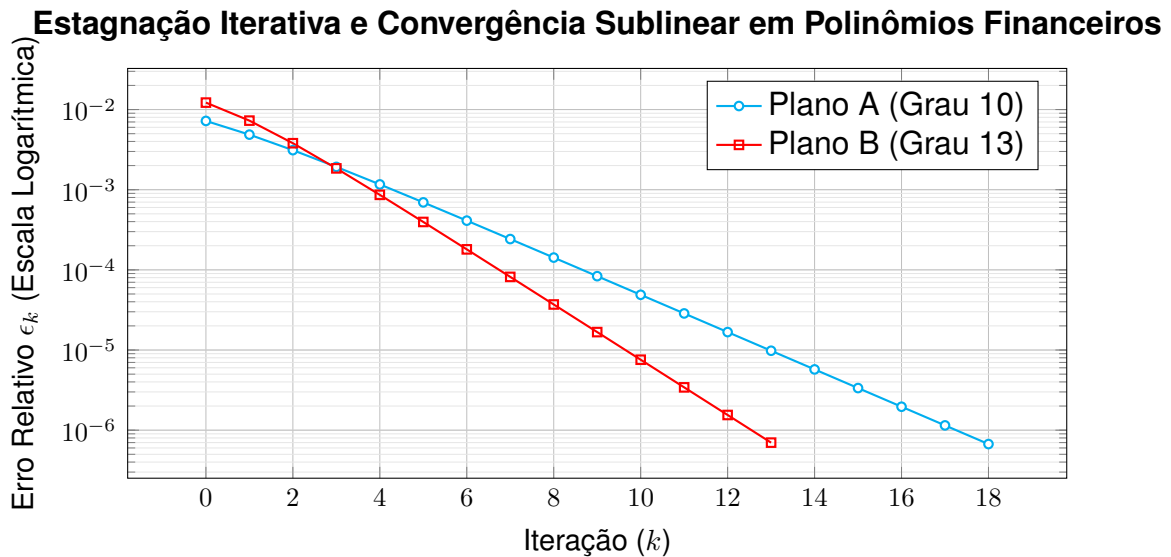
Figura 1.6: Convergência lenta da Posição Falsa prejudicada pela convexidade dos planos.
