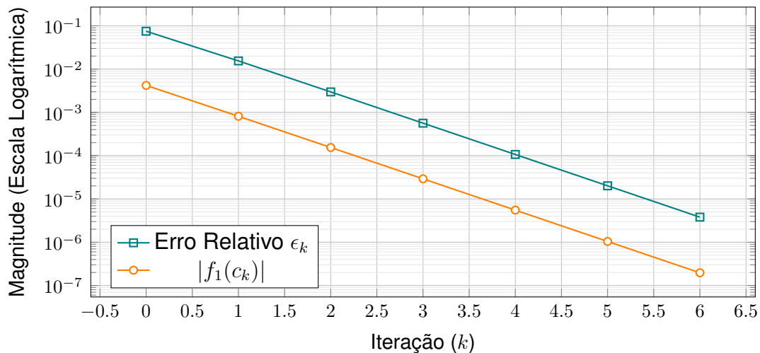
Figura 1.4: Amortecimento do erro e valor residual para f_1(T) .
