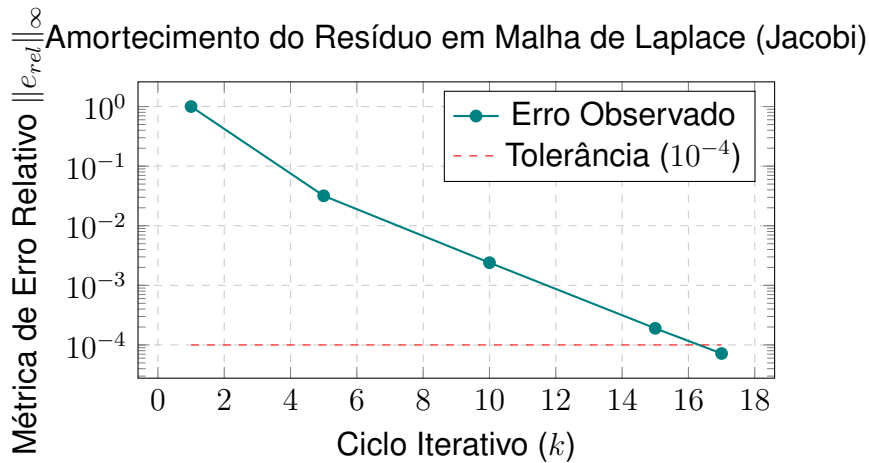
Figura 2.3: Amortecimento do Resíduo em Malha de Laplace (Jacobi)
