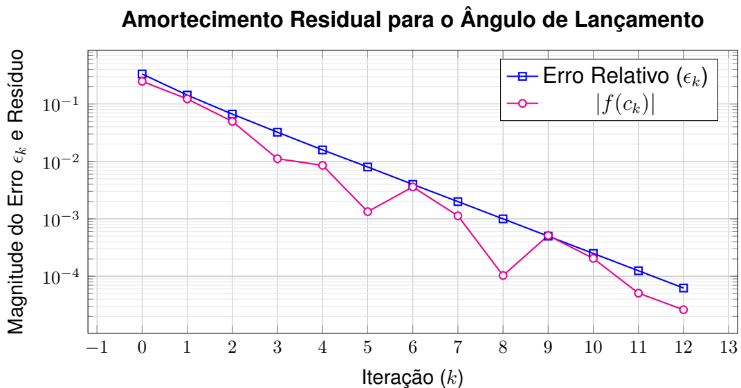
Figura 1.2: Convergência linear na busca de \alpha (Problema 3.6).
