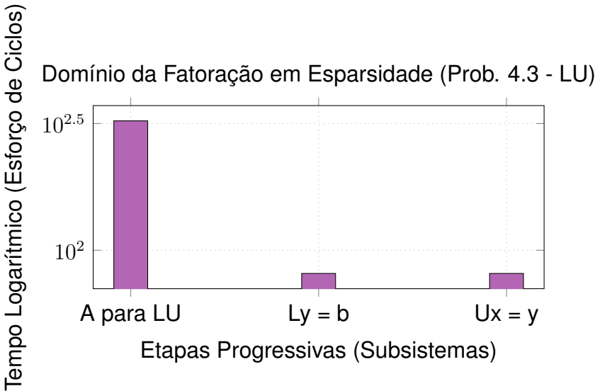
Figura 2.2: Domínio da Fatoração em Esparsidade (Prob. 4.3 - LU)
