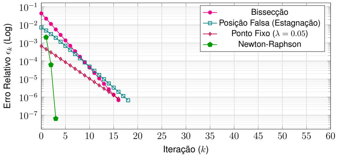
Figura 1.16: Visualização da penalidade imposta pela estagnação da Posição Falsa contraste com a convergência imediata da curva de Newton-Raphson.
