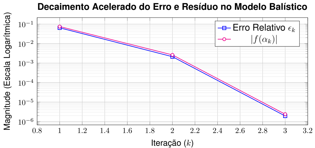
Figura 1.12: Convergência iterativa rápida de Newton-Raphson para prever \alpha .
