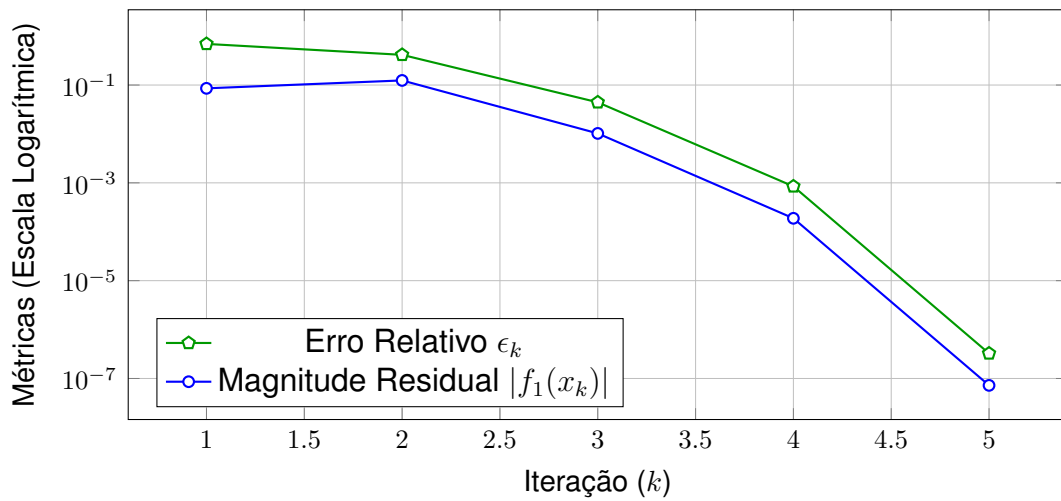
Figura 1.11: Amortecimento logarítmico demonstrando aceleração quadrática para f_1(T) .
