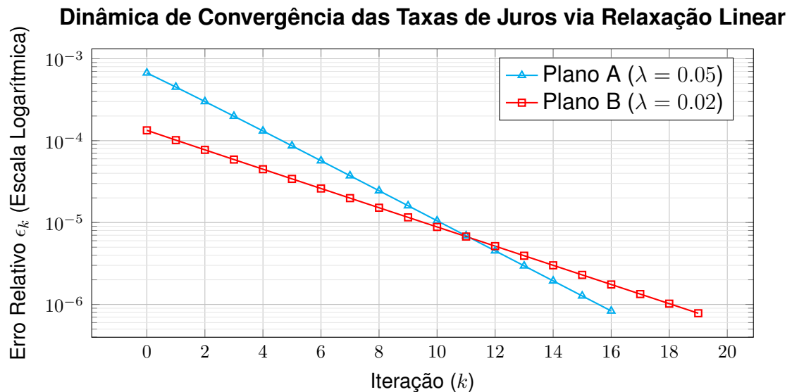
Figura 1.10: Convergência estável para a determinação de J_A e J_B .
