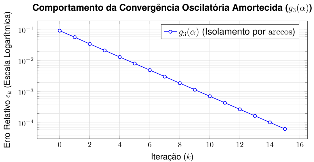
Figura 1.9: Decaimento do erro evidenciando a convergência linear para \alpha .
