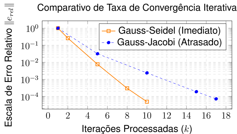
Figura 2.4: Comparativo de Taxa de Convergência Iterativa
