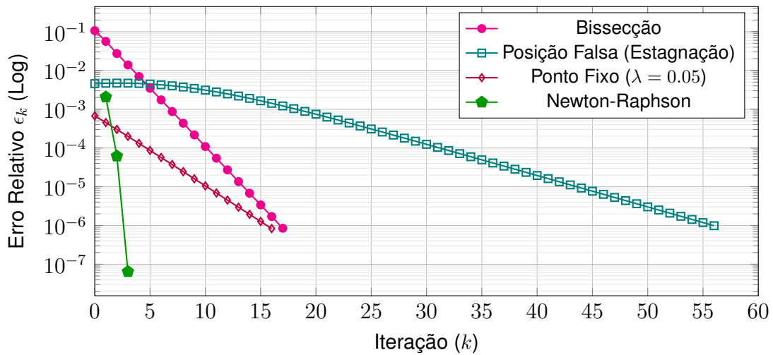
Figura 16: Visualização da penalidade imposta pela estagnação unilateral na Posição Falsa (arrasto até k = 56 ) em nítido contraste com o colapso imediato da curva de Newton-Raphson.
