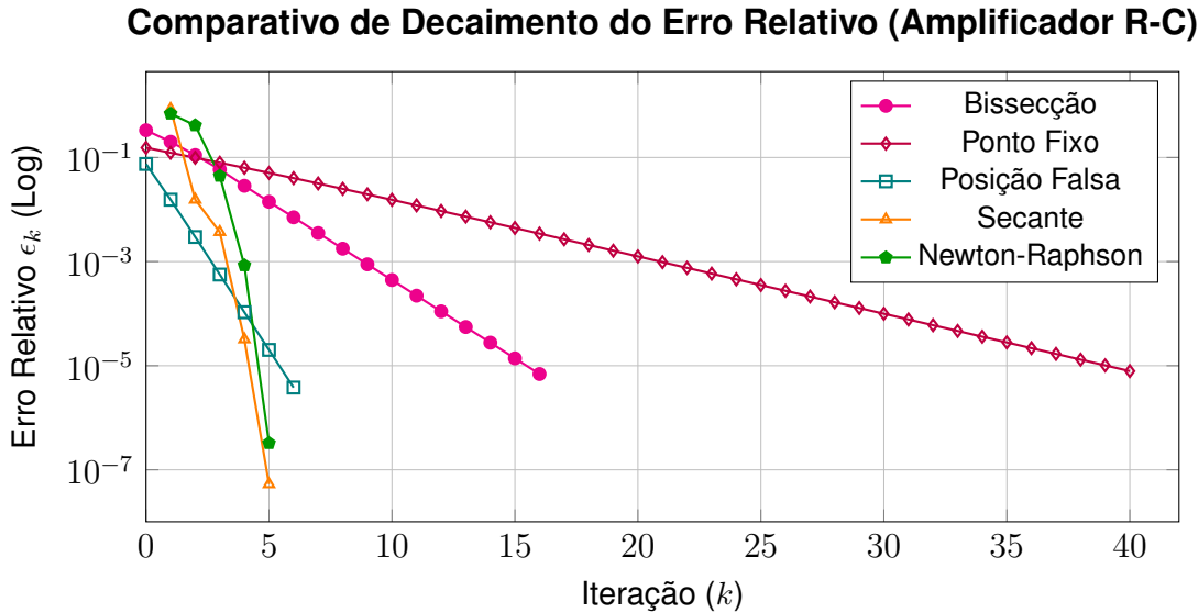
Figura 15: Superposição vetorial das taxas de convergência. O contraste entre a reta longa do Ponto Fixo ( \mathcal{O}(N) ) e a inflexão abrupta (concavidade para baixo) do Método de Newton reflete geometricamente as distintas ordens assintóticas.
