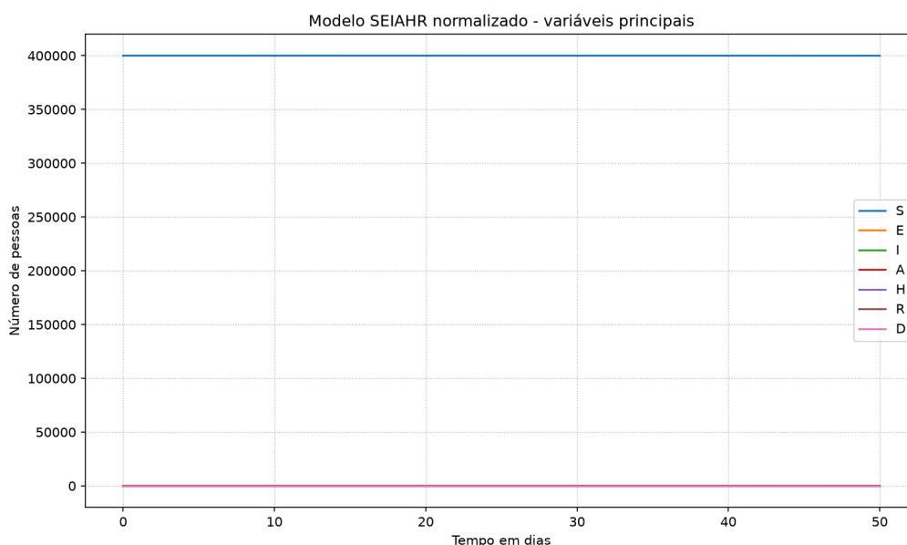
Figura 5: Evolução das variáveis do modelo SEIAHR normalizado.
