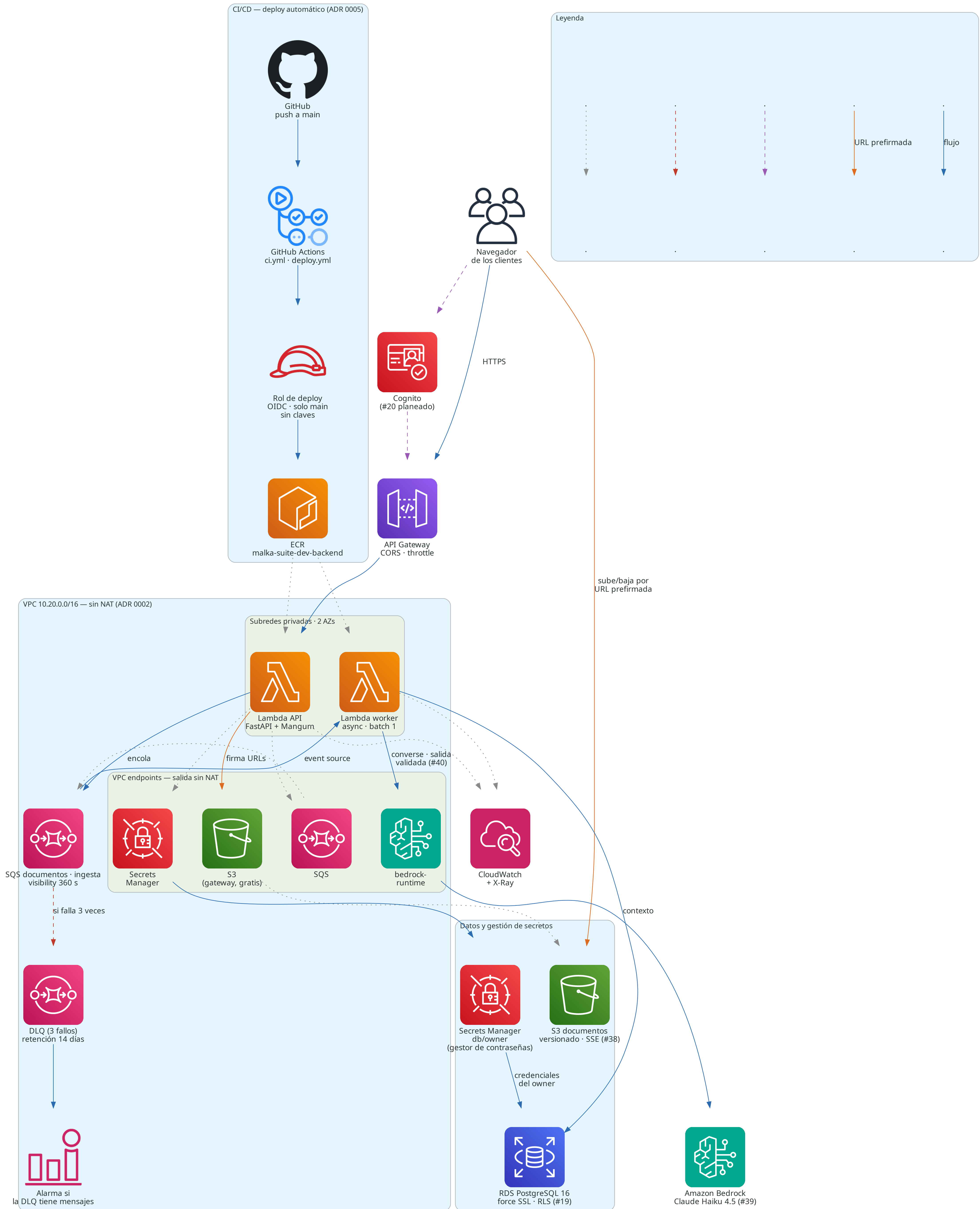
Malka Suite — arquitectura en AWS
