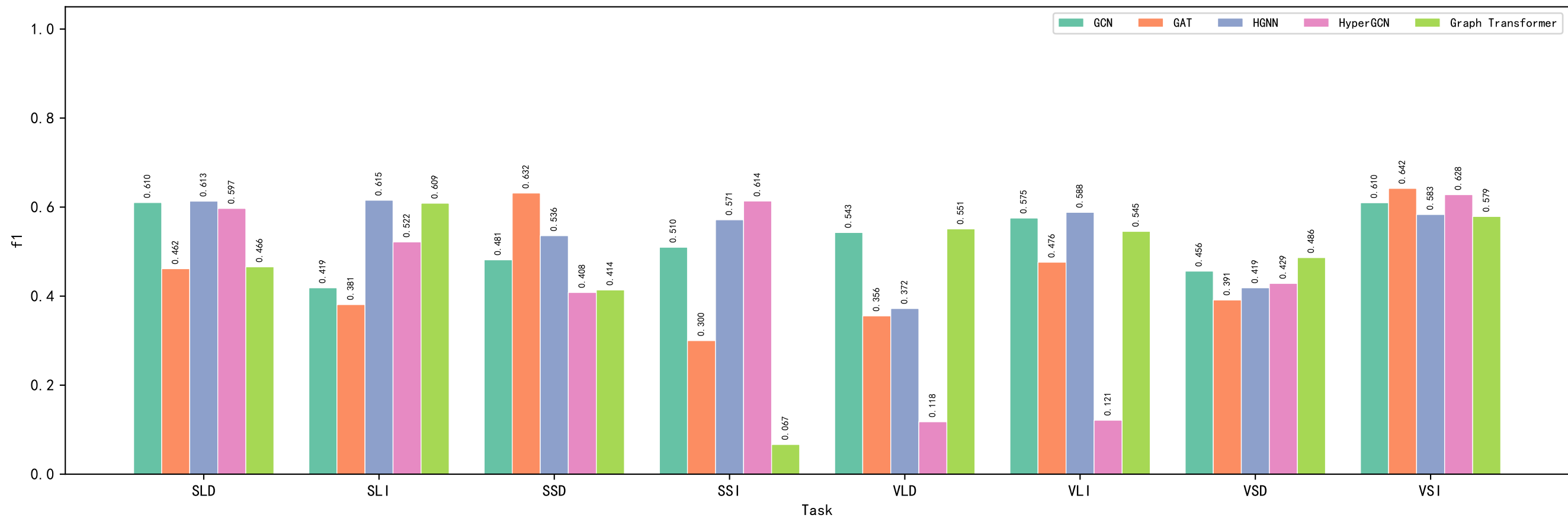
Model Comparison — f1
