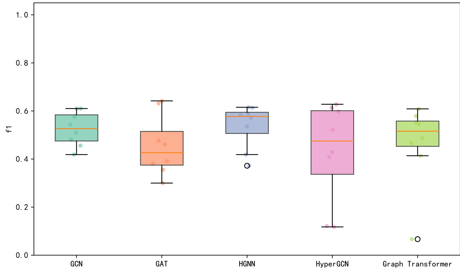
Performance Distribution — f1
