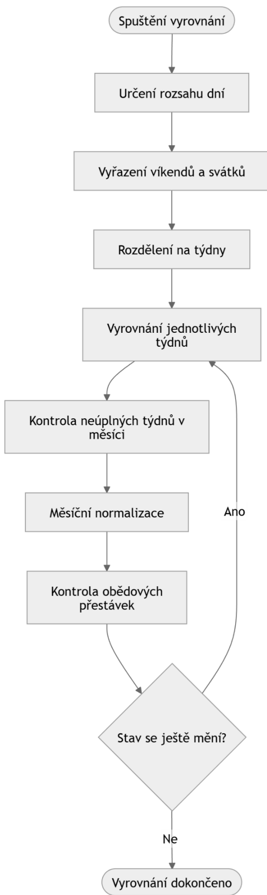
Obrázek 24 Celkový průběh algoritmu vyrovnávání hodin
