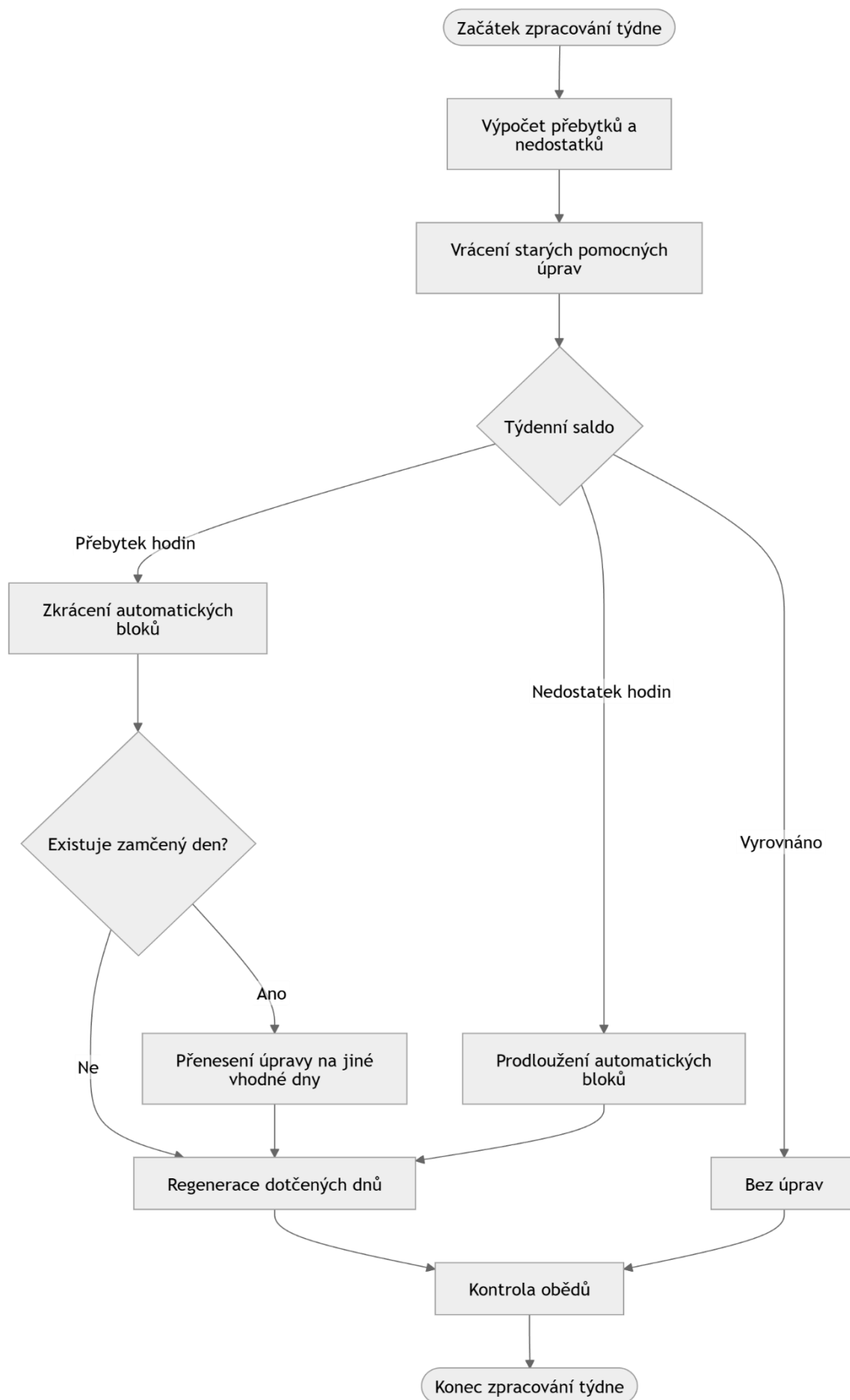
Obrázek 25 Zjednodušené schéma týdenního vyrovnání pracovní doby
