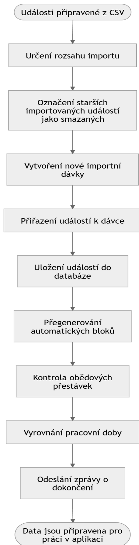
Obrázek 28 Uložení importovaných dat a navazující zpracování evidence
