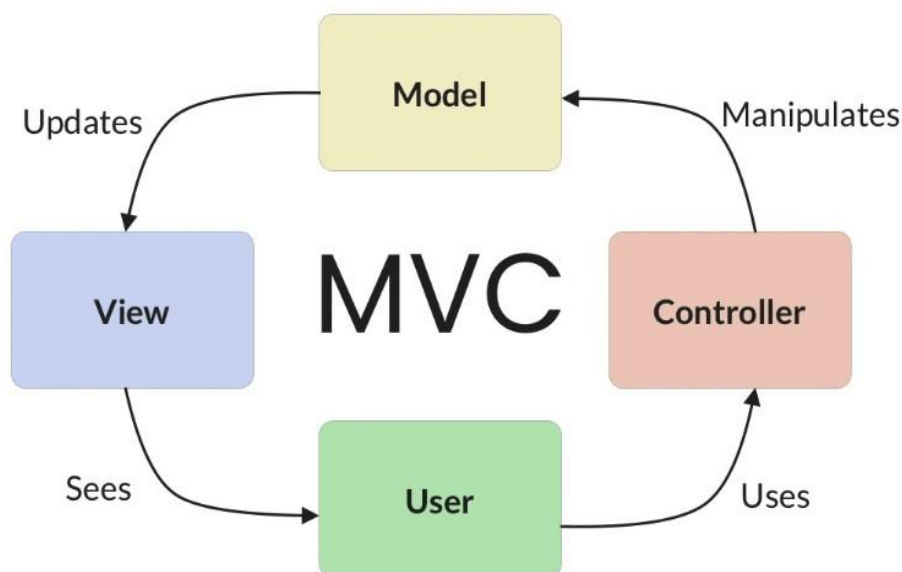
Obrázek 2 Architektura MVC
