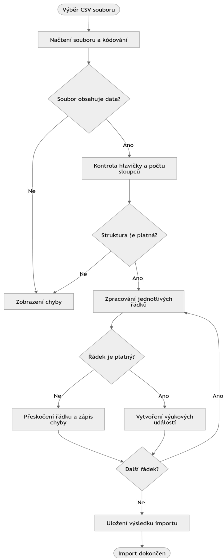
Obrázek 27 Základní průběh importu rozvrhu ze systému STAG
