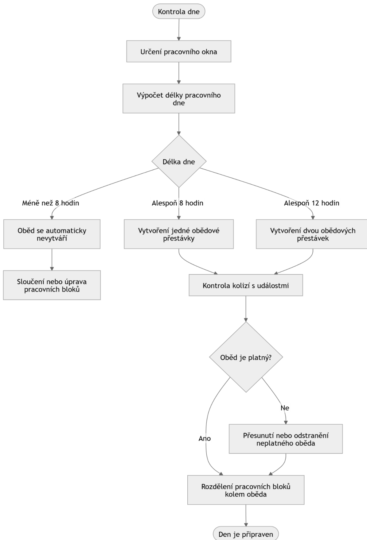
Obrázek 26 Kontrola a vytváření obědových přestávek
