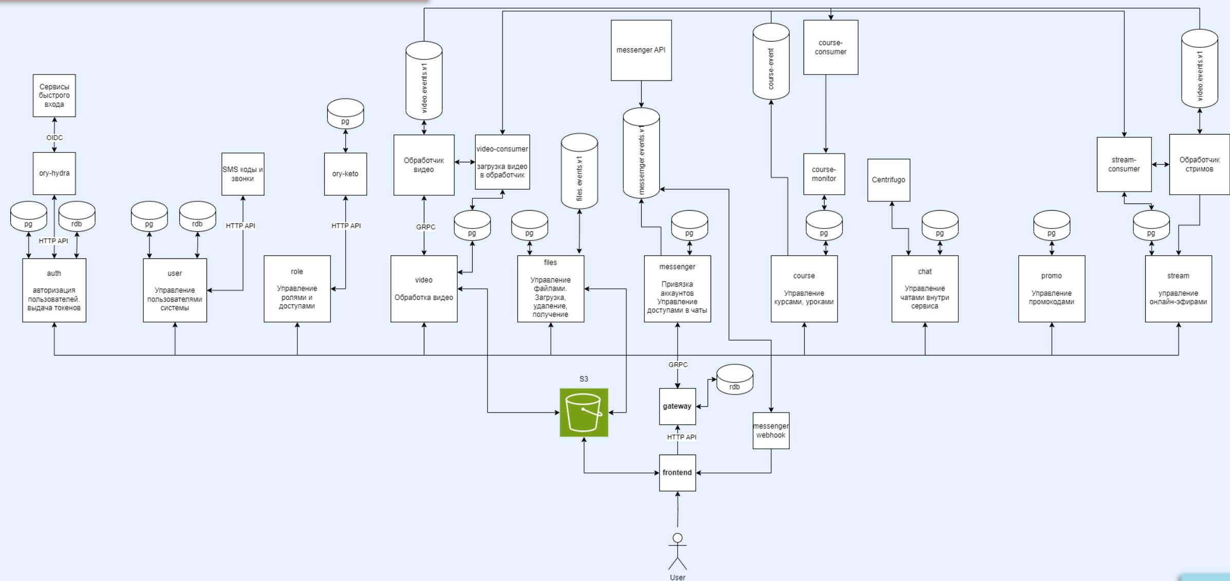
Рис. 2 – Архитектура проекта
