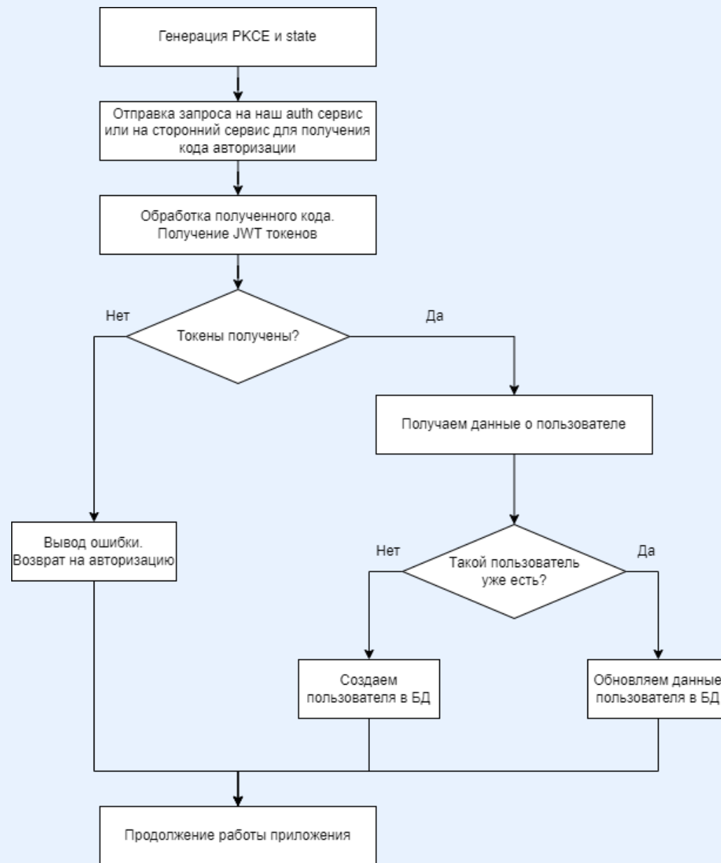
Рис. 3 – Блок-схема авторизации пользователя
