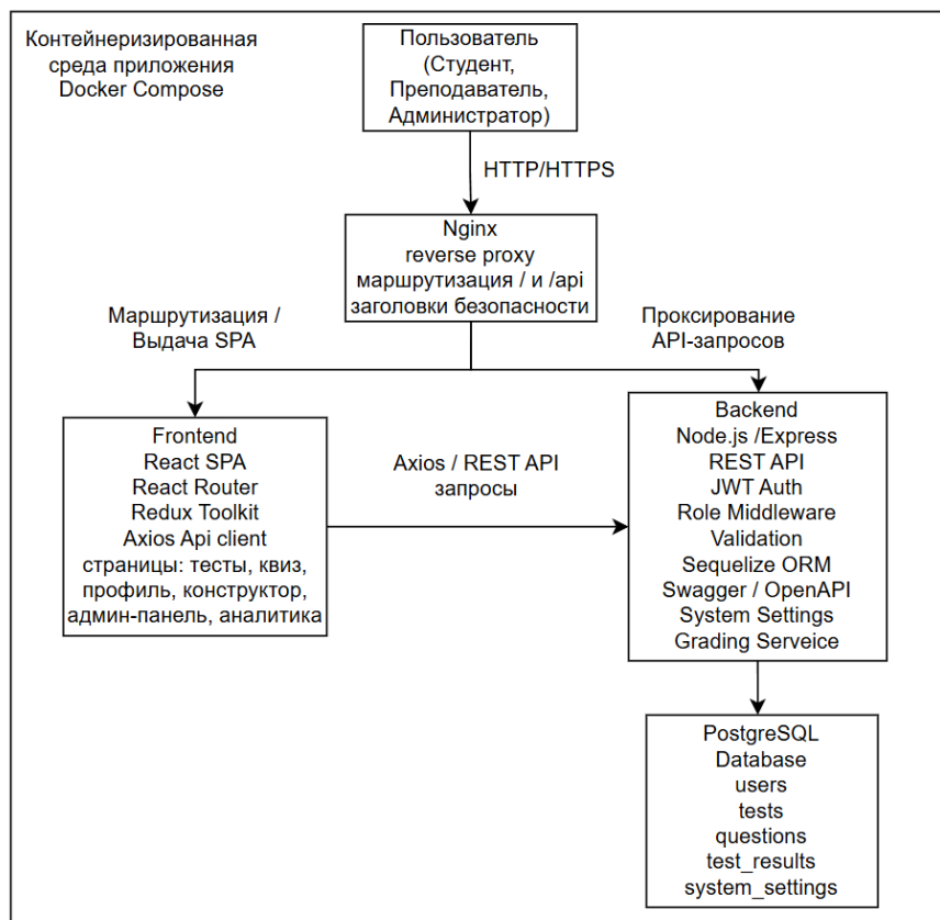
Рисунок 4 - Общая архитектура приложения «Интерактивный конструктор образовательных тестов»
