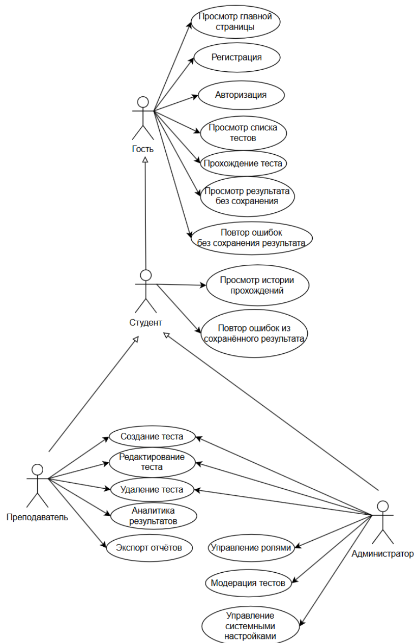
Рисунок 1 - UML-диаграмма вариантов использования
