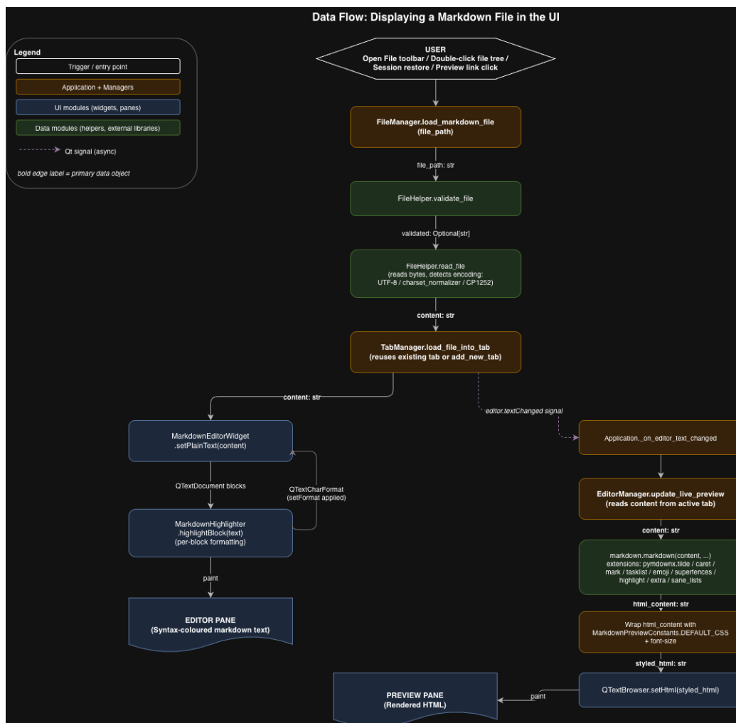
Obrázek 3: Tok dat při zobrazení markdown souboru: FileManager využívá FileHelper k validaci a načtení obsahu, TabManager obsluhuje záložky a editor; živý náhled vzniká převodem markdownu na HTML a zobrazením v náhledovém widgetu.
