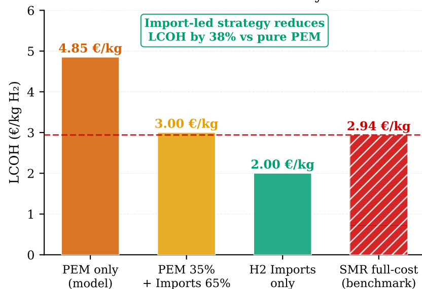
(d) Decarbonisation options for Eni Sannazzaro refinery
