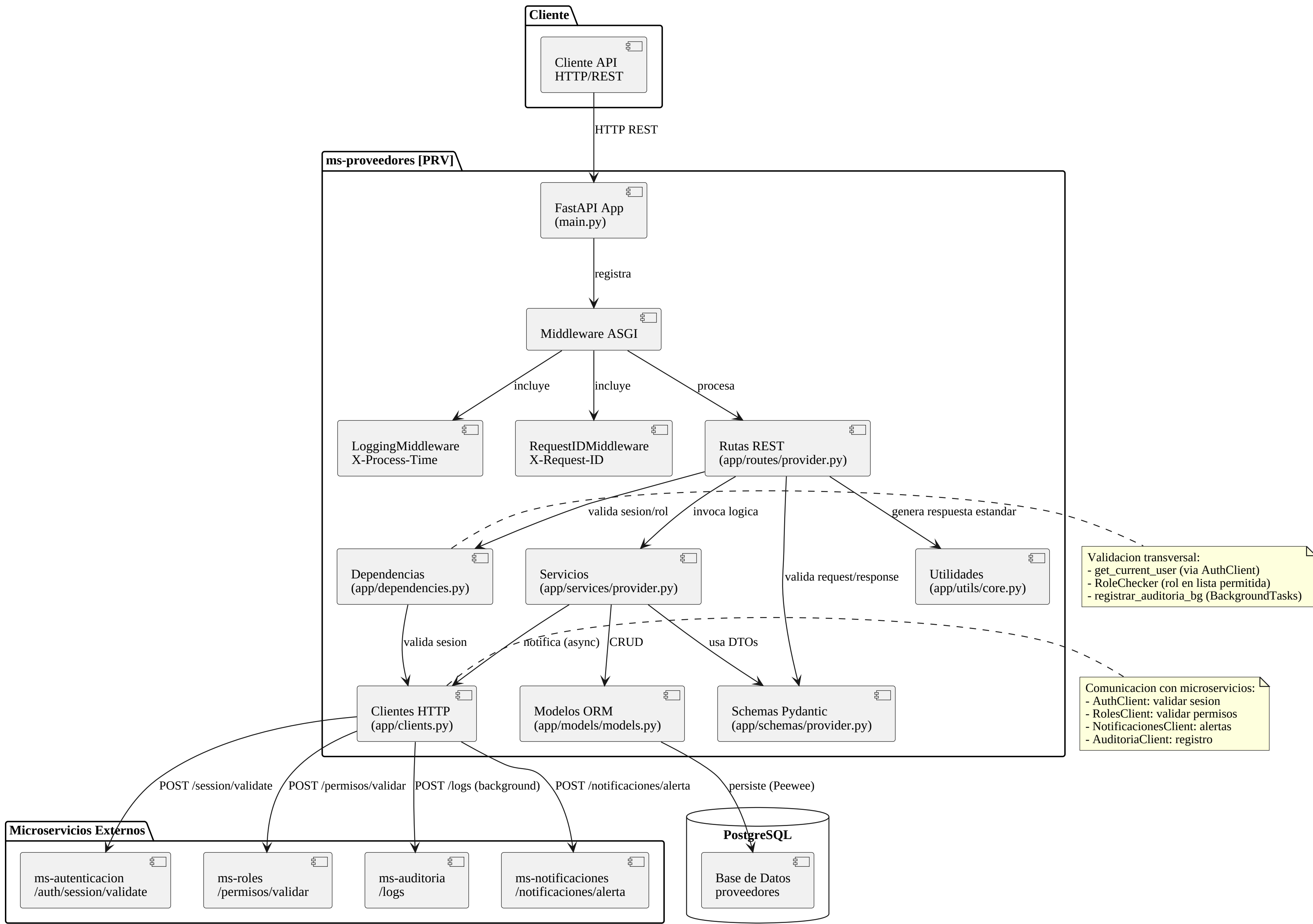
Diagrama de Componentes — ms-proveedores [PRV]
