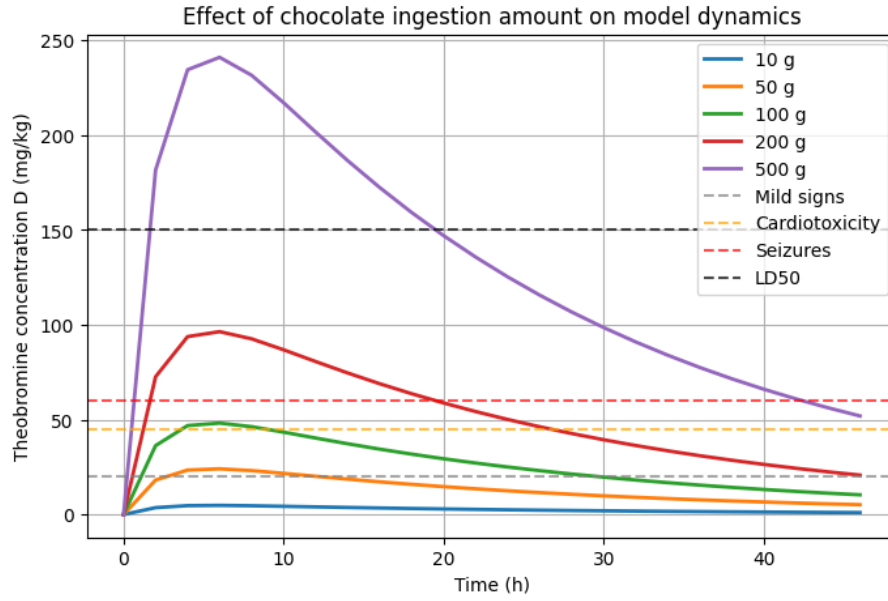
Figure 4: Effets de la quantité de chocolat ingéré sur la dynamique du modèle.
